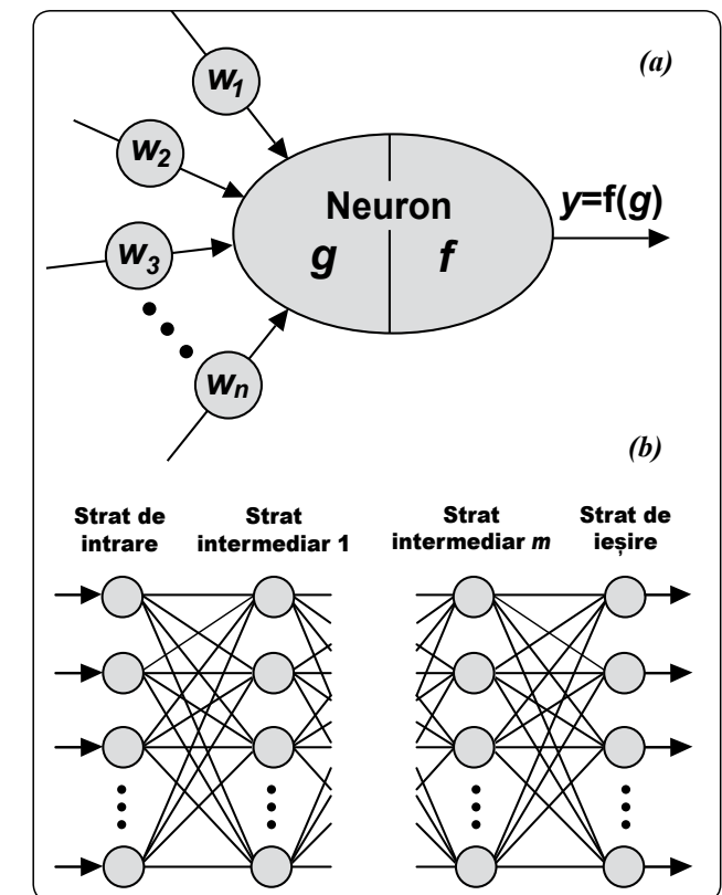
Fig. 10. Neuron artificial (a) și rețea neuronală multistrat (b) formare (testarea preciziei modelului folosind o serie diferită de componente pentru a recunoaște datele inițiale); recunoaș-
